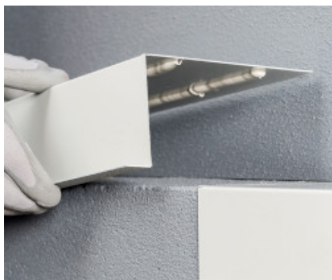
Incollaggio elastico di elementi costruttivi
