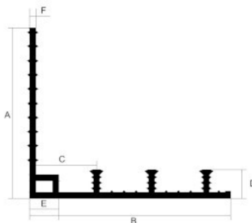
Idrostop PVC KR
